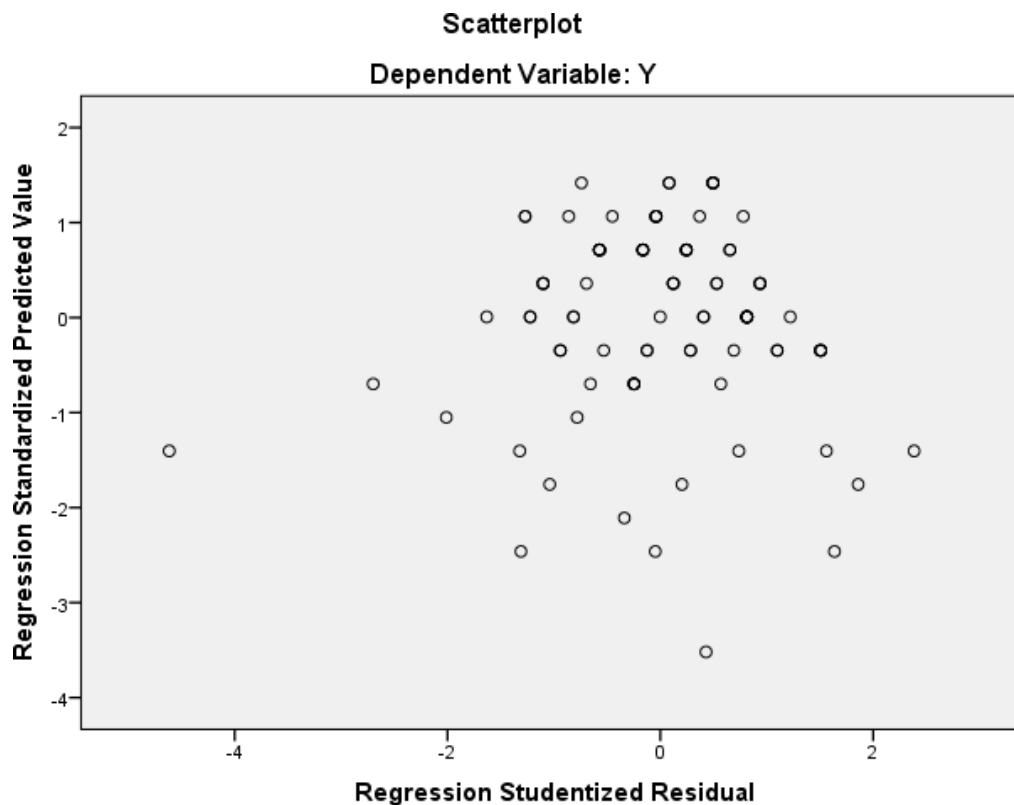
Gambar 1 Grafik Scatterplot
